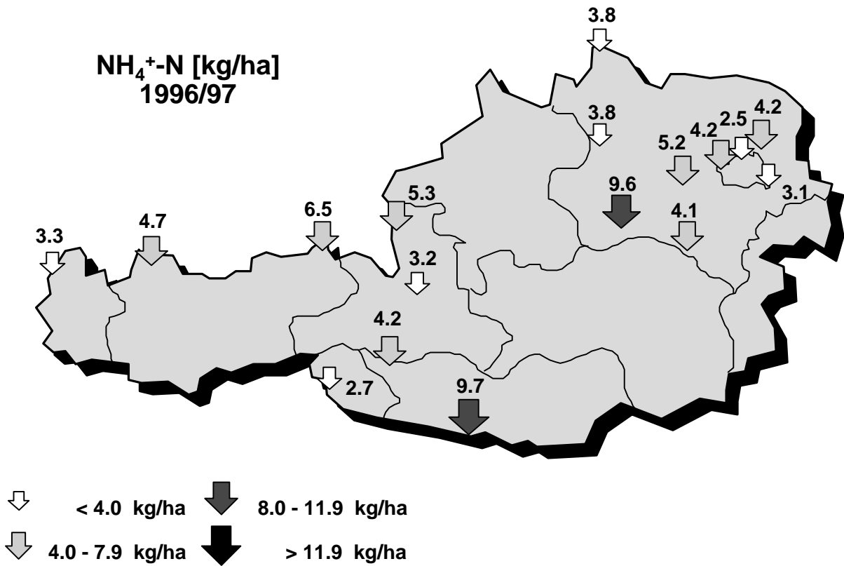
Abb.3a,b: Räumliche Verteilung der mengengewichteten NH 4 + -N Jahreskonzentrationen im Niederschlag sowie der NH 4 + -N Einträge für den Zeitraum Oktober 1996 bis September 1997 (für Hard: April 1996 bis März 1997)
