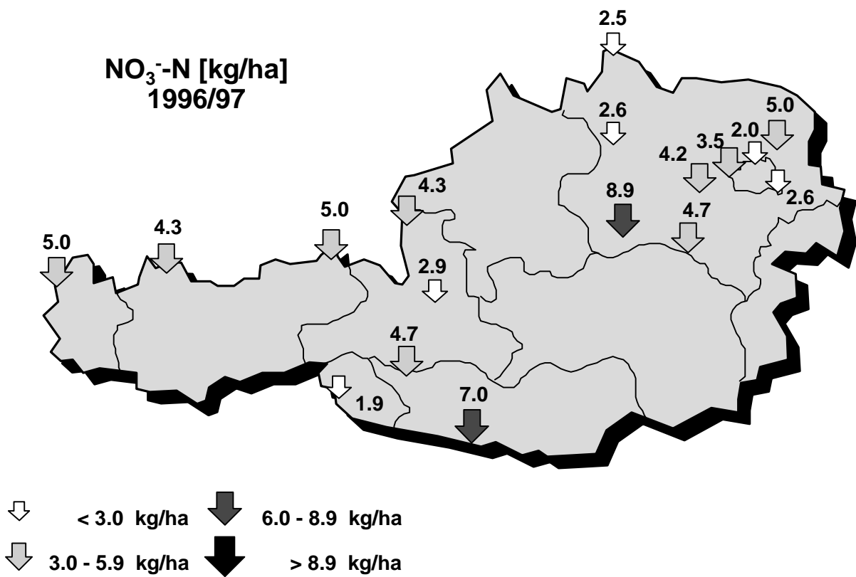
Abb.4a,b: Räumliche Verteilung der mengengewichteten NO 3 - -N Jahreskonzentrationen im Niederschlag sowie der NO 3 - -N Einträge für den Zeitraum Oktober 1996 bis September 1997 (für Hard: April 1996 bis März 1997)
