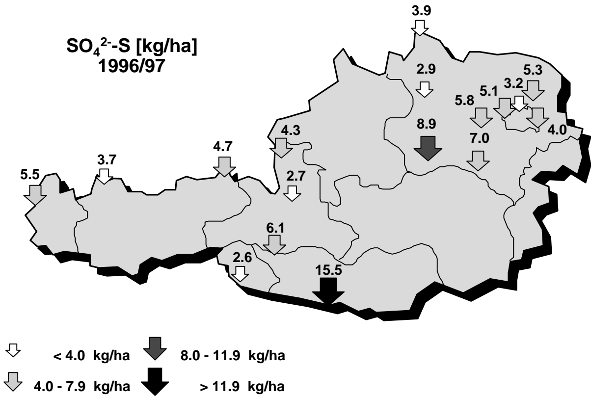
Abb.2a,b: Räumliche Verteilung der mengengewichteten SO 4 2- -S Jahreskonzentrationen im Niederschlag sowie der SO 4 2- -S Einträge für den Zeitraum Oktober 1996 bis September 1997 (für Hard: April 1996 bis März 1997)
