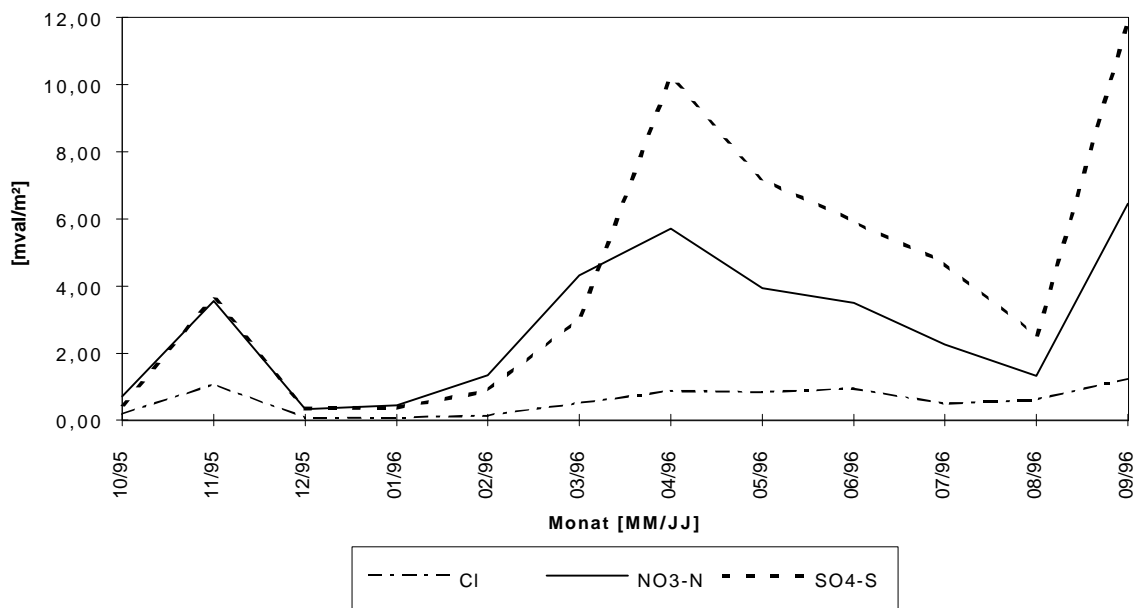
Abb.6a: Zeitreihe der monatlichen Kationen- und Anioneneinträge für den Zeitraum Oktober 1995 bis September 1996 an der Station: Naßwald
