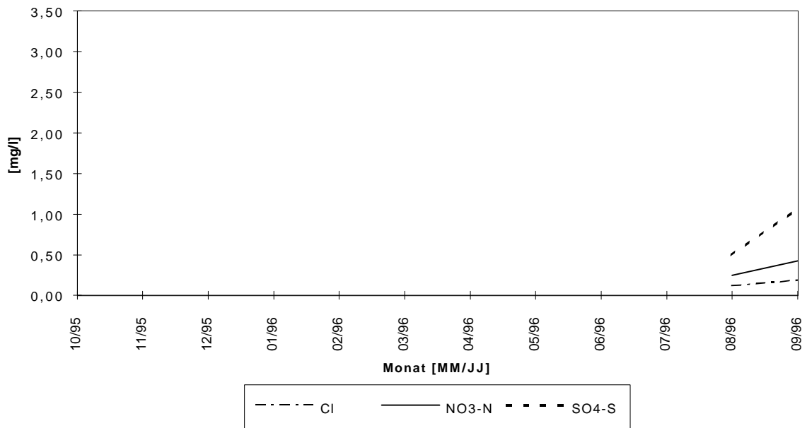
Abb.5b: Zeitreihe der monatlichen Kationen- und Anionenkonzentrationen im Niederschlag für den Zeitraum Oktober 1995 bis September 1996 an der Station: Lainz
