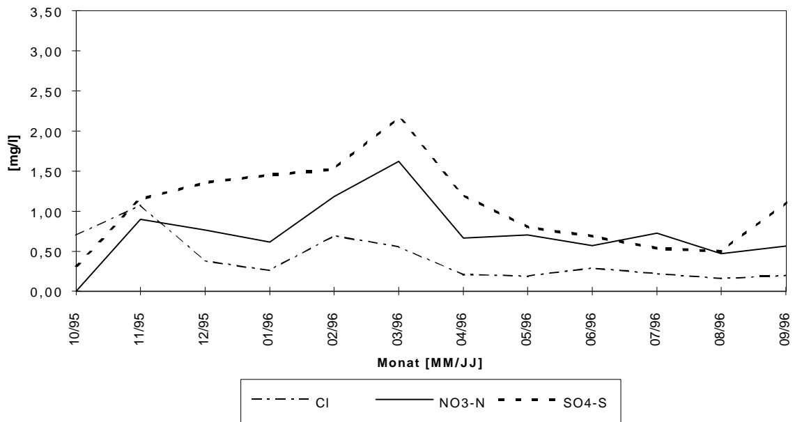
Abb.5c: Zeitreihe der monatlichen Kationen- und Anionenkonzentrationen im Niederschlag für den Zeitraum Oktober 1995 bis September 1996 an der Station: Lobau
