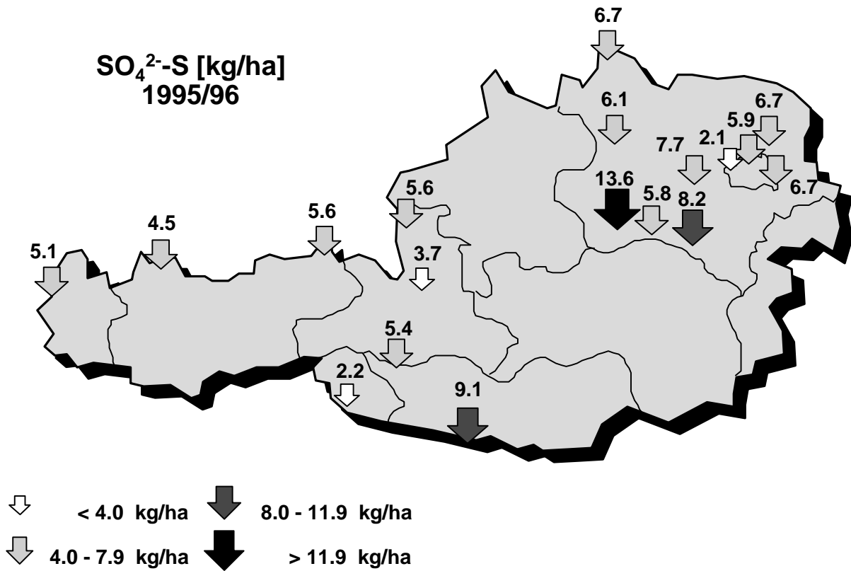
Abb.2a,b: Räumliche Verteilung der mengengewichteten SO 4 2- -S Jahreskonzentrationen im Niederschlag sowie der SO 4 2- -S Einträge für den Zeitraum Oktober 1995 bis September 1996 (für Hard: April 1995 bis März 1996)
