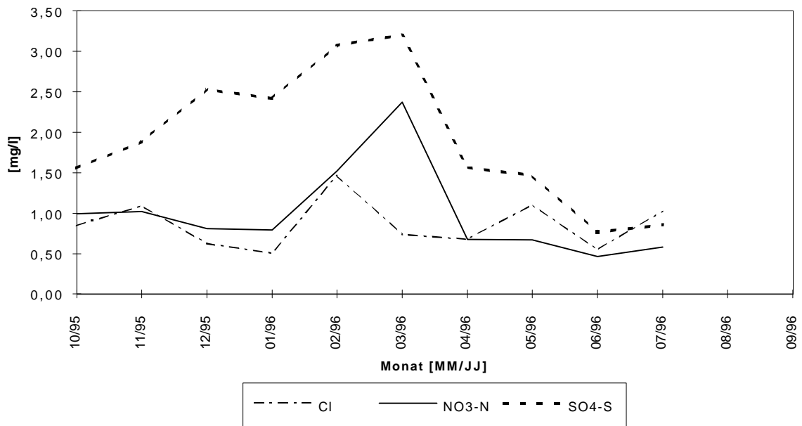
Abb.5d: Zeitreihe der monatlichen Kationen- und Anionenkonzentrationen im Niederschlag für den Zeitraum Oktober 1995 bis September 1996 an der Station: Bisamberg
