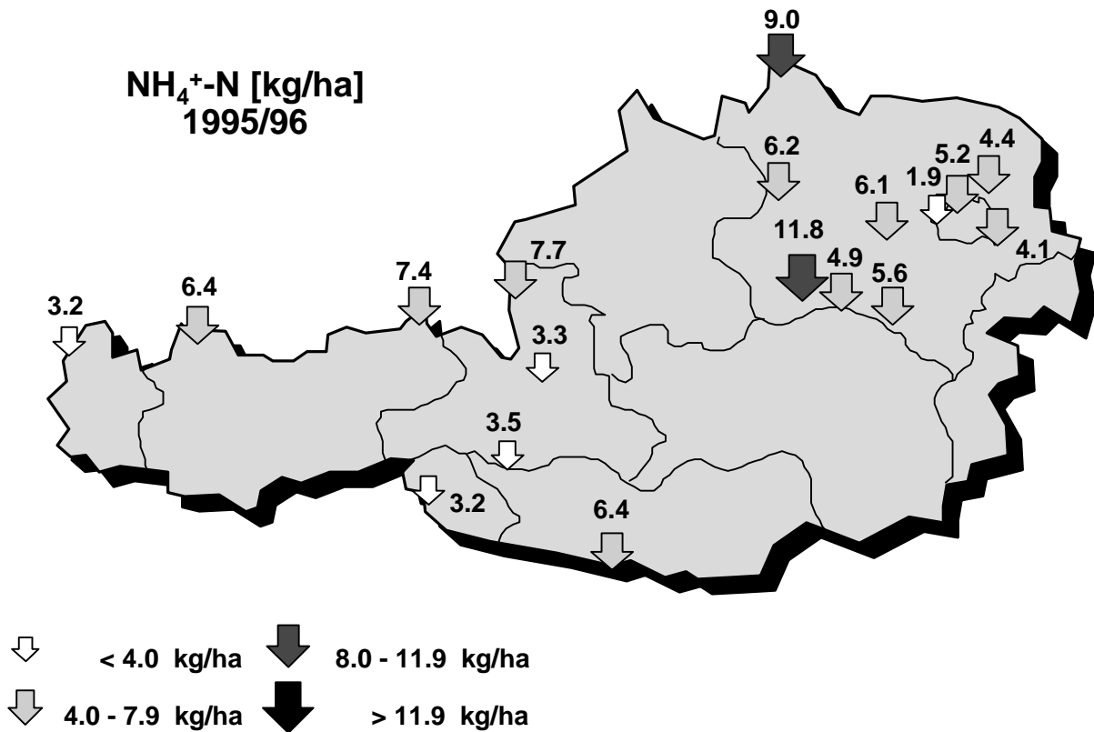
Abb.3a,b: Räumliche Verteilung der mengengewichteten NH 4 + -N Jahreskonzentrationen im Niederschlag sowie der NH 4 + -N Einträge für den Zeitraum Oktober 1995 bis September 1996 (für Hard: April 1995 bis März 1996)
