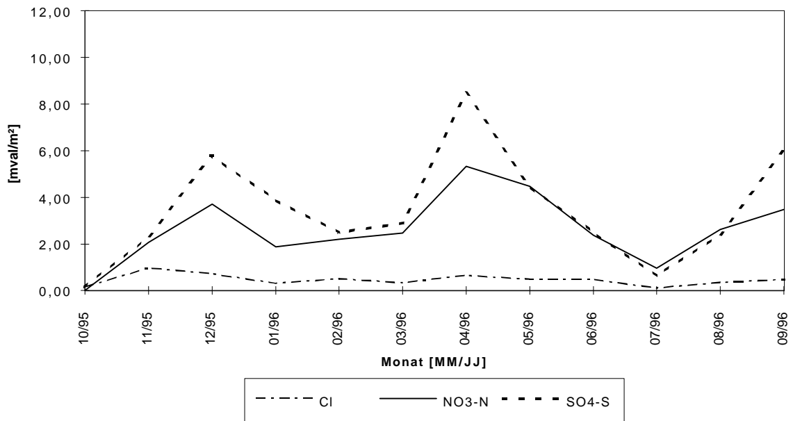
Abb.6c: Zeitreihe der monatlichen Kationen- und Anioneneinträge für den Zeitraum Oktober 1995 bis September 1996 an der Station: Lobau
