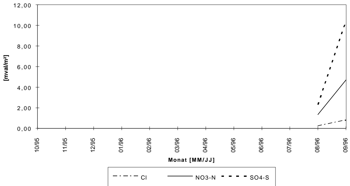
Abb.6b: Zeitreihe der monatlichen Kationen- und Anioneneinträge für den Zeitraum Oktober 1995 bis September 1996 an der Station: Lainz
