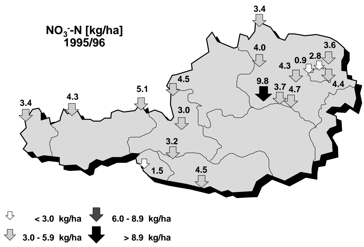
Abb.4a,b: Räumliche Verteilung der mengengewichteten NO 3 - -N Jahreskonzentrationen im Niederschlag sowie der NO 3 - -N Einträge für den Zeitraum Oktober 1995 bis September 1996 (für Hard: April 1995 bis März 1996)
