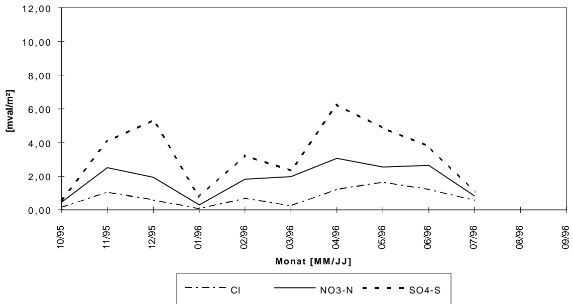
Abb.6d: Zeitreihe der monatlichen Kationen- und Anioneneinträge für den Zeitraum Oktober 1995 bis September 1996 an der Station: Bisamberg
