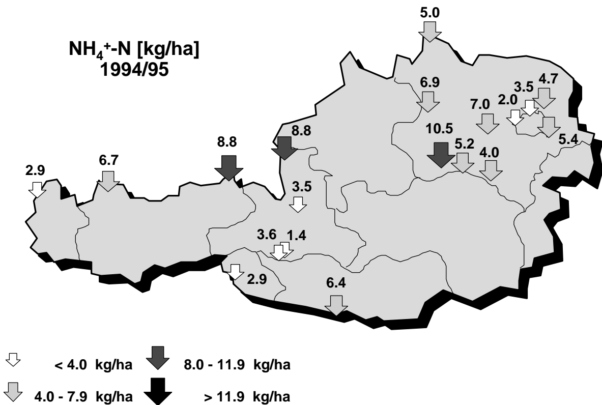
Abb.3a,b: Räumliche Verteilung der mengengewichteten NH 4 + -N Jahreskonzentrationen im Niederschlag sowie der NH 4 + -N Einträge für den Zeitraum Oktober 1994 bis September 1995 (für Hard: Mai 1994 bis März 1995)
