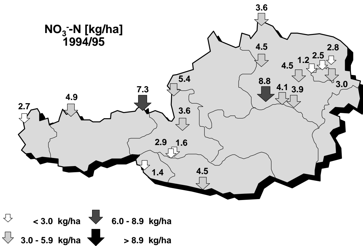
Abb.4a,b: Räumliche Verteilung der mengengewichteten NO 3 - -N Jahreskonzentrationen im Niederschlag sowie der NO 3 - -N Einträge für den Zeitraum Oktober 1994 bis September 1995 (für Hard: Mai 1994 bis März 1995)
