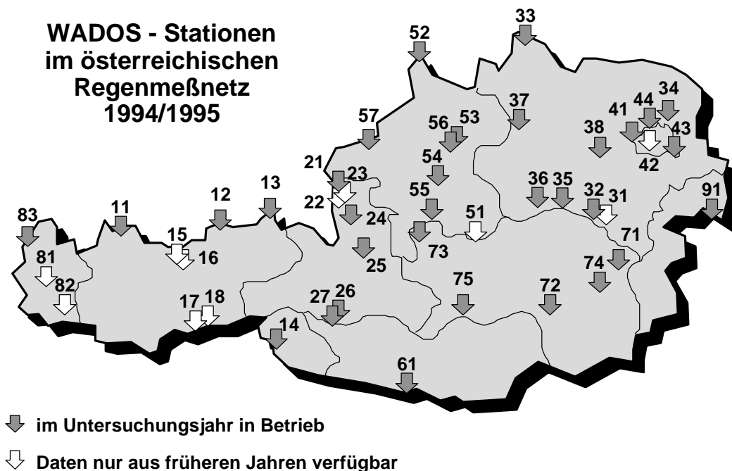
Abb.1: Lage der WADOS Stationen im österreichischen Niederschlagsmeßnetz für des Niederschlagsjahr 1994/95
