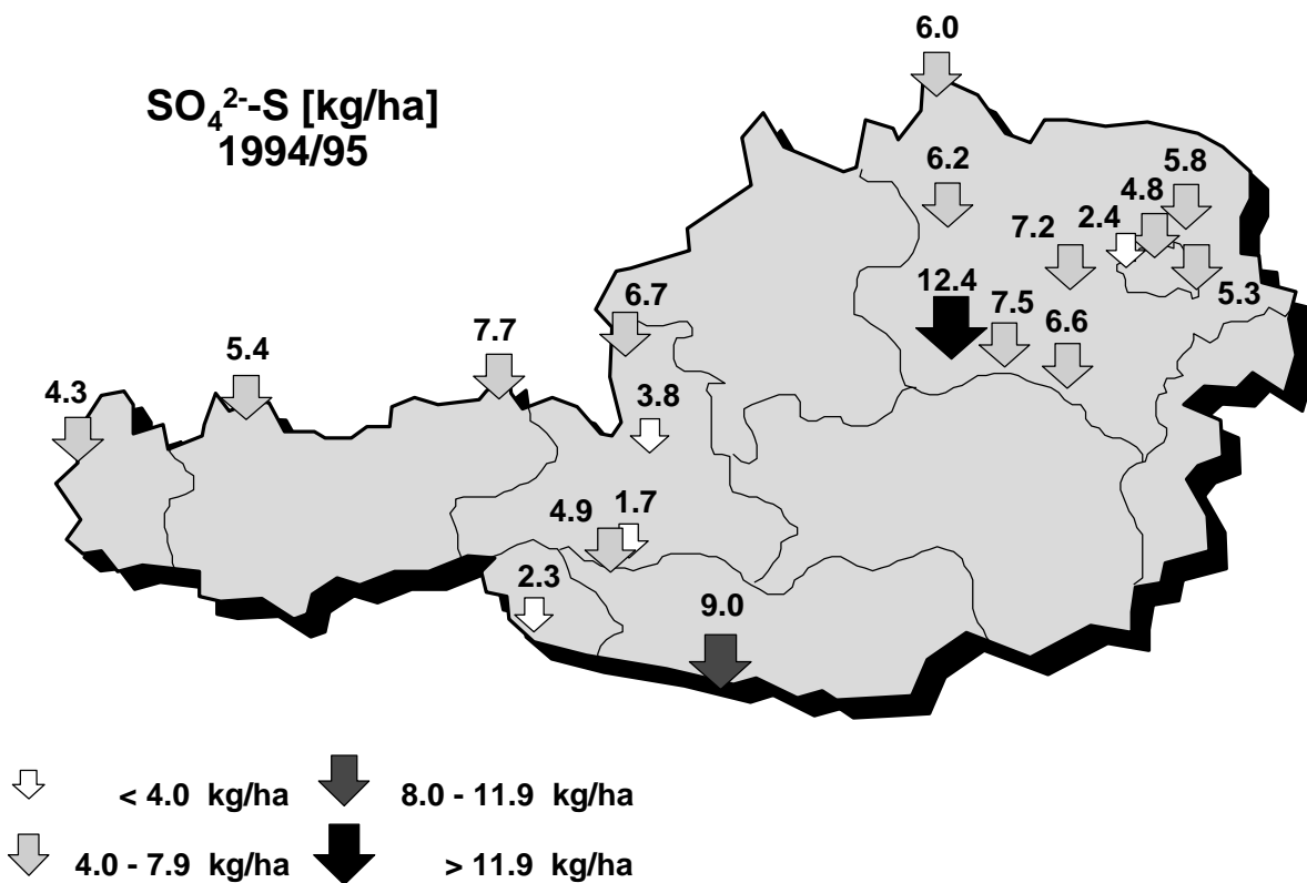
Abb.2a,b: Räumliche Verteilung der mengengewichteten SO 4 2- -S Jahreskonzentrationen im Niederschlag sowie der SO 4 2- -S Einträge für den Zeitraum Oktober 1994 bis September 1995 (für Hard: Mai 1994 bis März 1995)
